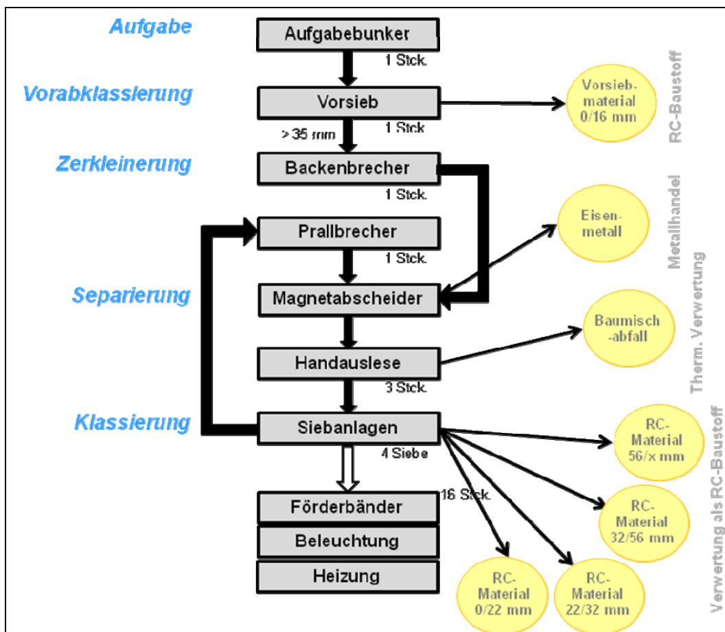
Abb. 29: Prozessübersicht Trockenaufbereitung 26
