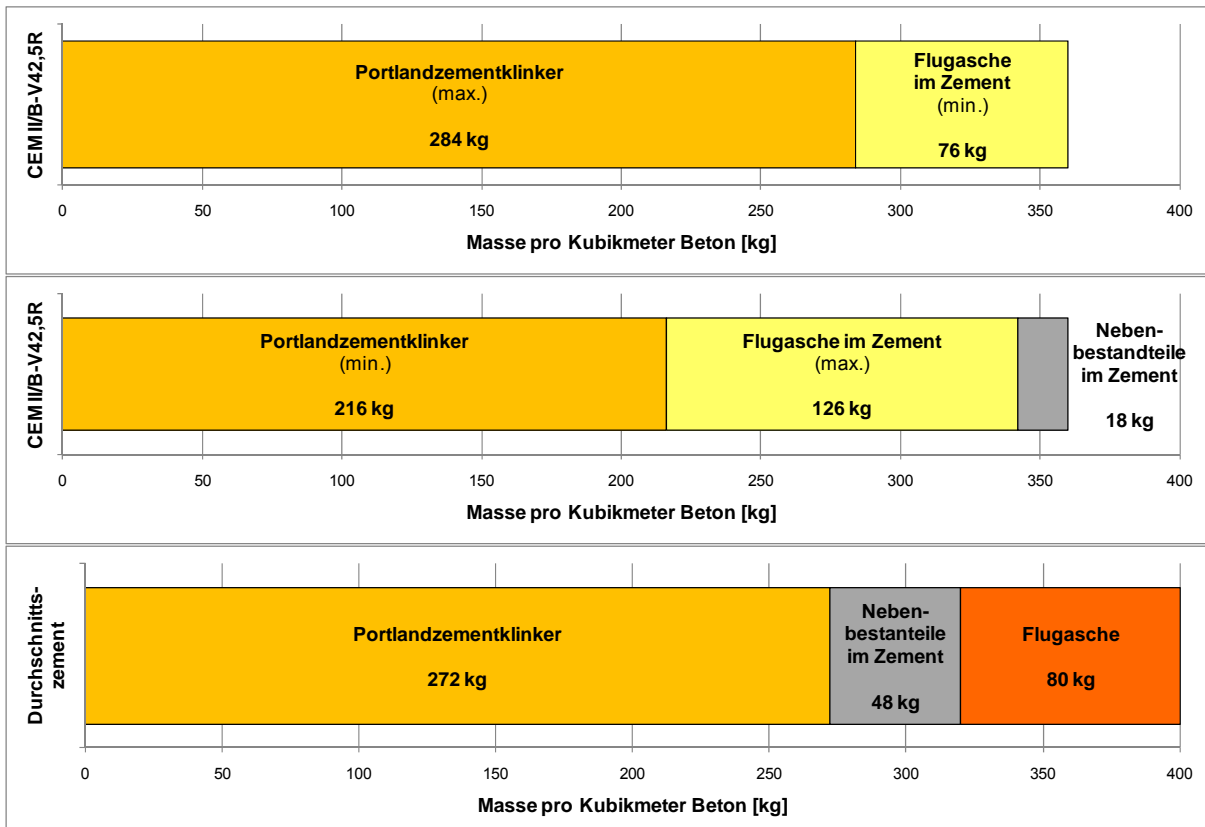
Abb. 20: Synopse der Bindemittelzusammensetzung von RC-Beton C 30/37, Vergleichsbeton C 30/37 (TBS) – CEM II/B-V42,5R und Standardbeton C 30/37 (BTB) – Durchschnittszement
