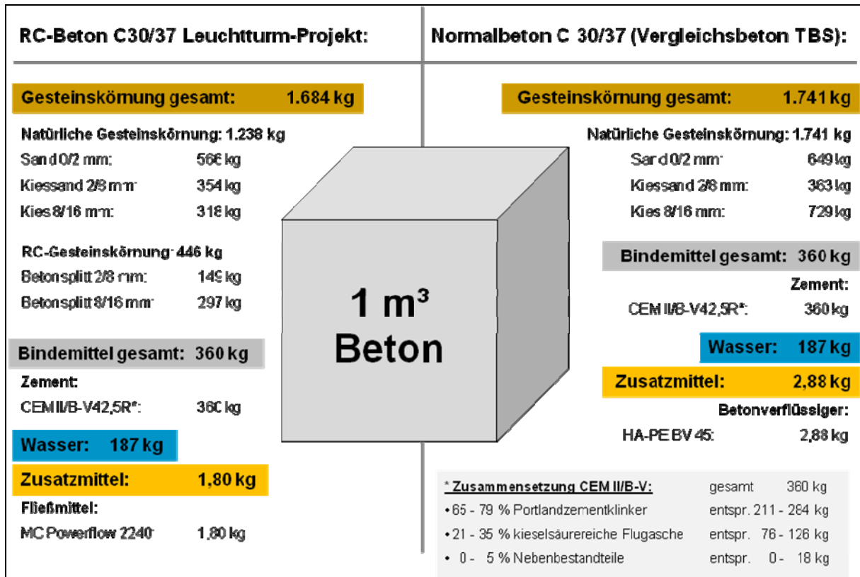
Abb. 16: Gegenüberstellung Ausgangsstoffe RC-Beton / Normalbeton C 30/37 der Fa. TBS 16
